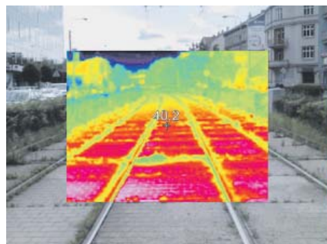
Termosnímek ulice, na jejíž části se nachází zelený tramvajový pás. Termokamera naměřila na zelené části trati 27 °C, na betonové části 40,2 °C. Rozdíl teplot tedy činí 13 °C. Hodnota 30 °C se navíc jeví jako zásadní, protože pokud se teplota zvýší nad tuto hranici, je ochlazování pro náš organismus náročné.
