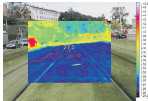
Termosnímek ulice, na jejíž části se nachází zelený tramvajový pás. Termokamera naměřila na zelené části trati 27 °C, na betonové části 40,2 °C. Rozdíl teplot tedy činí 13 °C. Hodnota 30 °C se navíc jeví jako zásadní, protože pokud se teplota zvýší nad tuto hranici, je ochlazování pro náš organismus náročné.
